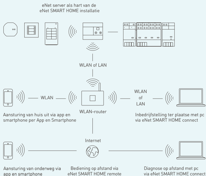
eNet server – overzicht
