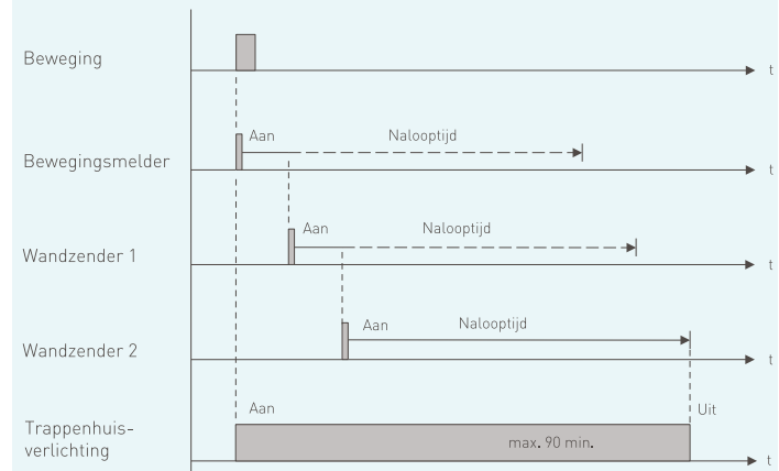
Werkingsprincipe trappenhuisverlichtingsschakeling
