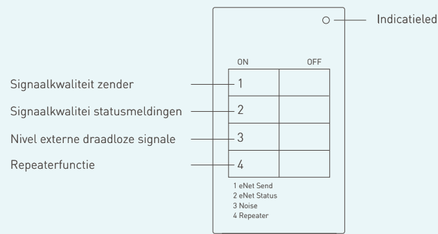
eNet diagnose-apparaat
