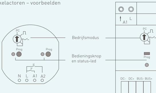
Schakelactoren – voorbeelden
