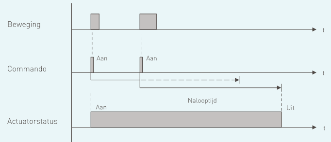
Werkingsprincipe eNet bewegingsmelding
